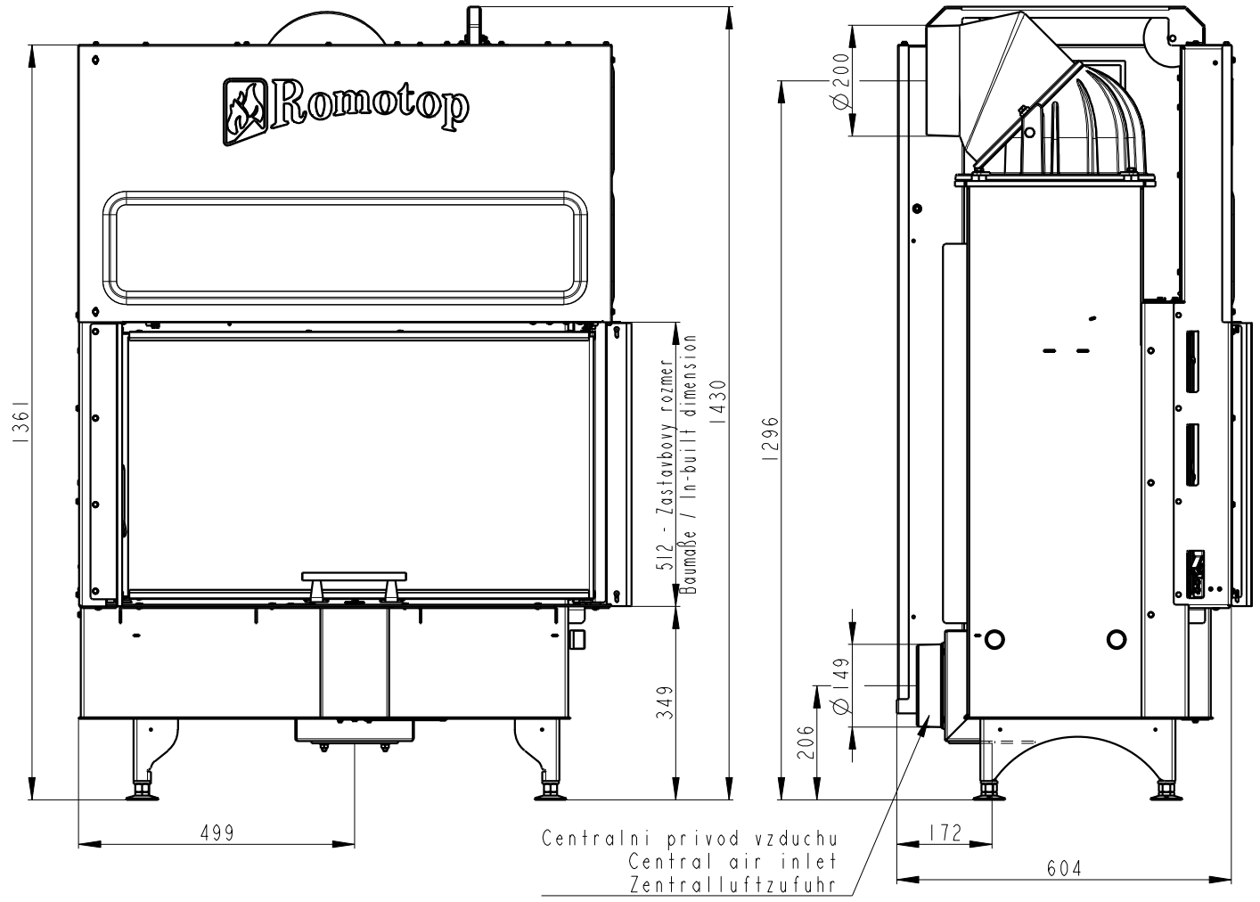
Otocna kopule s kolenom Cast iron turning dome Rotierende Kuppel mit Knie
