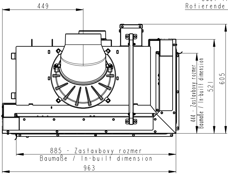
Primarni a sekundarni vzduch Primärluft und Sekundärluft Primary and secondary air
